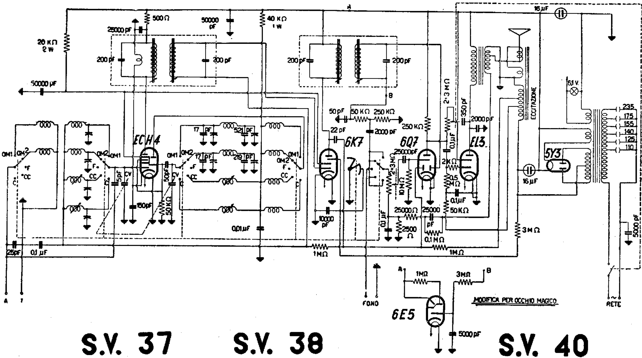
MAGNADYNE RADIO - Modelli SV 37, SV 38, SV 40, SV 140 RADIOFONOGRFO - Lo schema corrisponde anche al mod. SV 18, senza 6E5. Gamma onde medie divisa, due gamme onde corte. Due reazioni negative, dal secondario del trasformatore d'uscita e dalla placca della EL3. Media frequenza 471,5 kc/s. Potenza d'uscita 4 W. Consumo 60 W.
